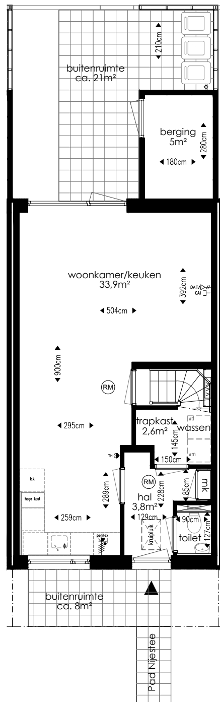
Begane grond
